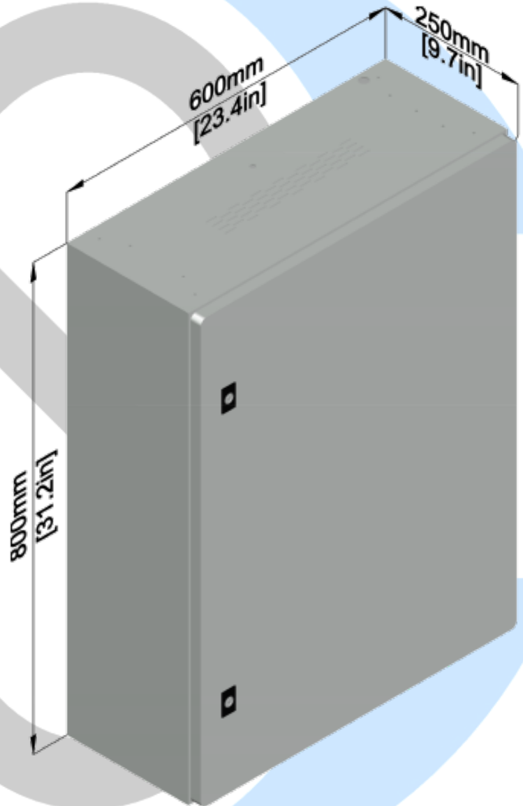
Cotas Armario C MR Eléctricos VVVF
