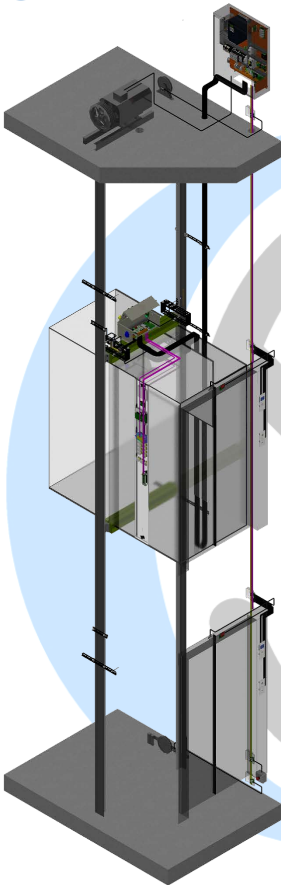
Ubicación Armario C MR en Instalaciones Eléctricas con cuarto de Máquinas
